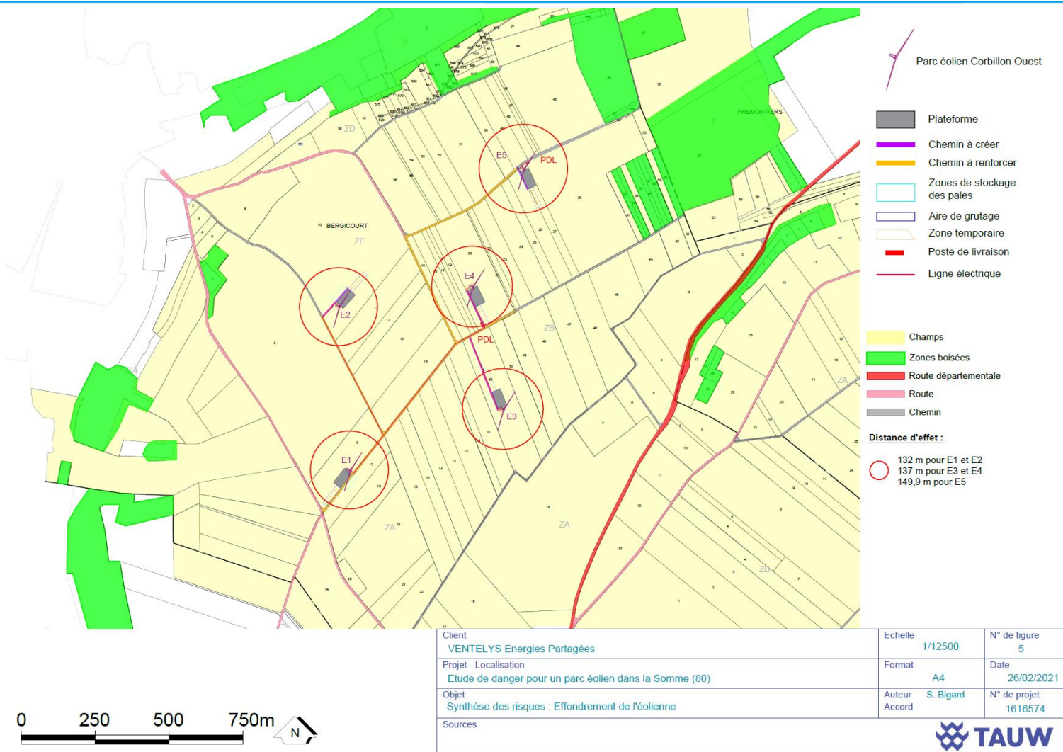
Figure 14 : Effondrement de l'éolienne – carte des distances d'effets
