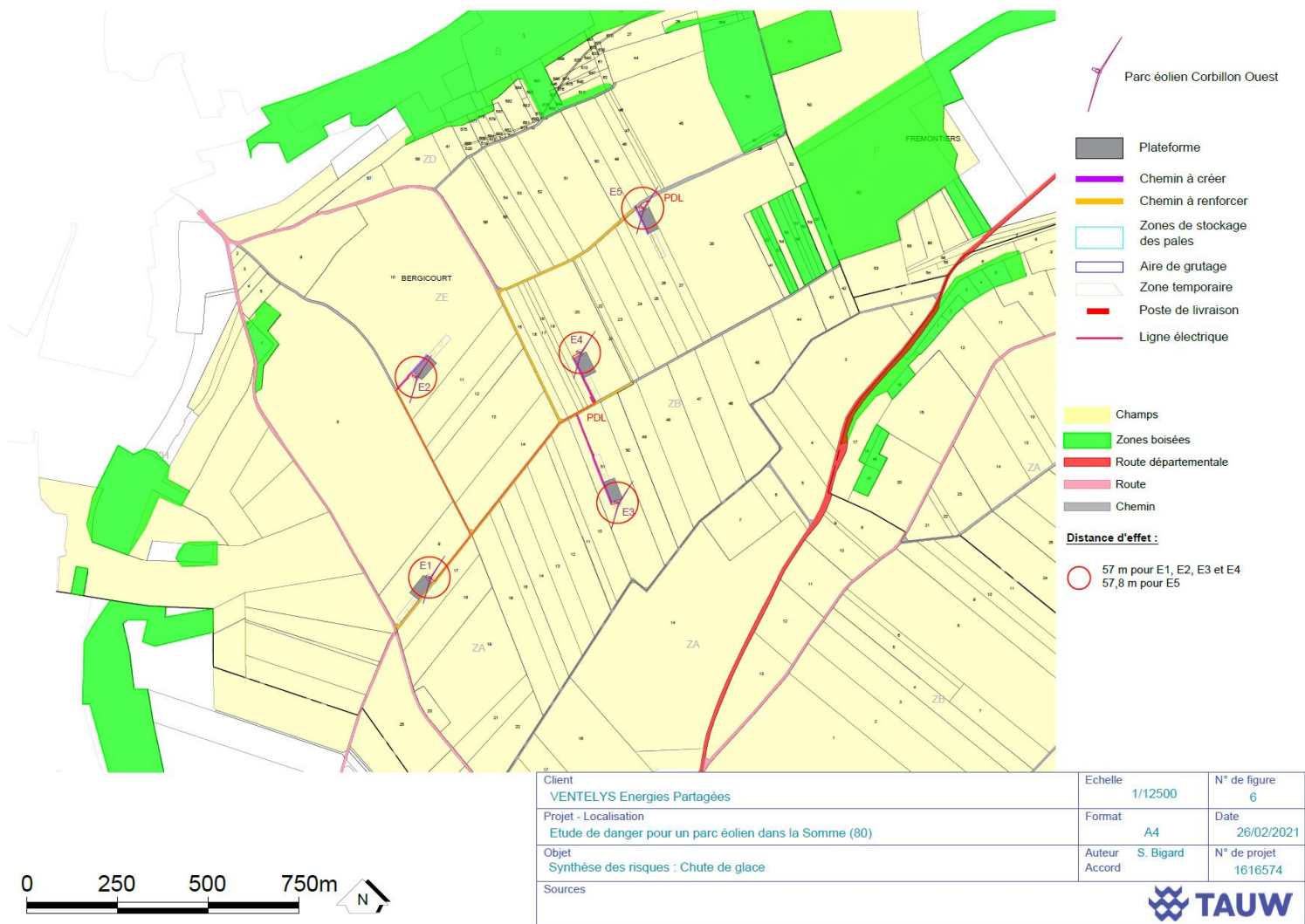
Figure 16 : Chute de glace – carte des distances d'effets
